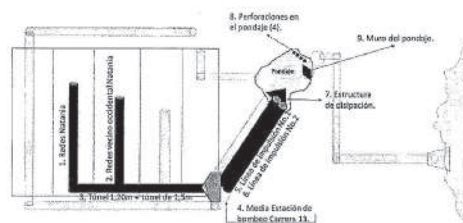
Esquema Ejecución Fase 1
