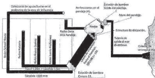
Figura 2. Esquema de los componentes del sistema, bajo las condiciones inicialmente viabilizadas
