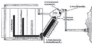
Figura 2. Esquema del componente alcantarillado pluvial SAI ETAPA 1.
